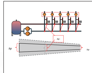
混合回路供暖系统
