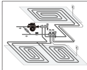
地板采暖系统
