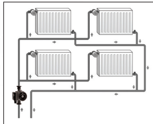
双管供热系统
