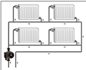
单管供热系统
