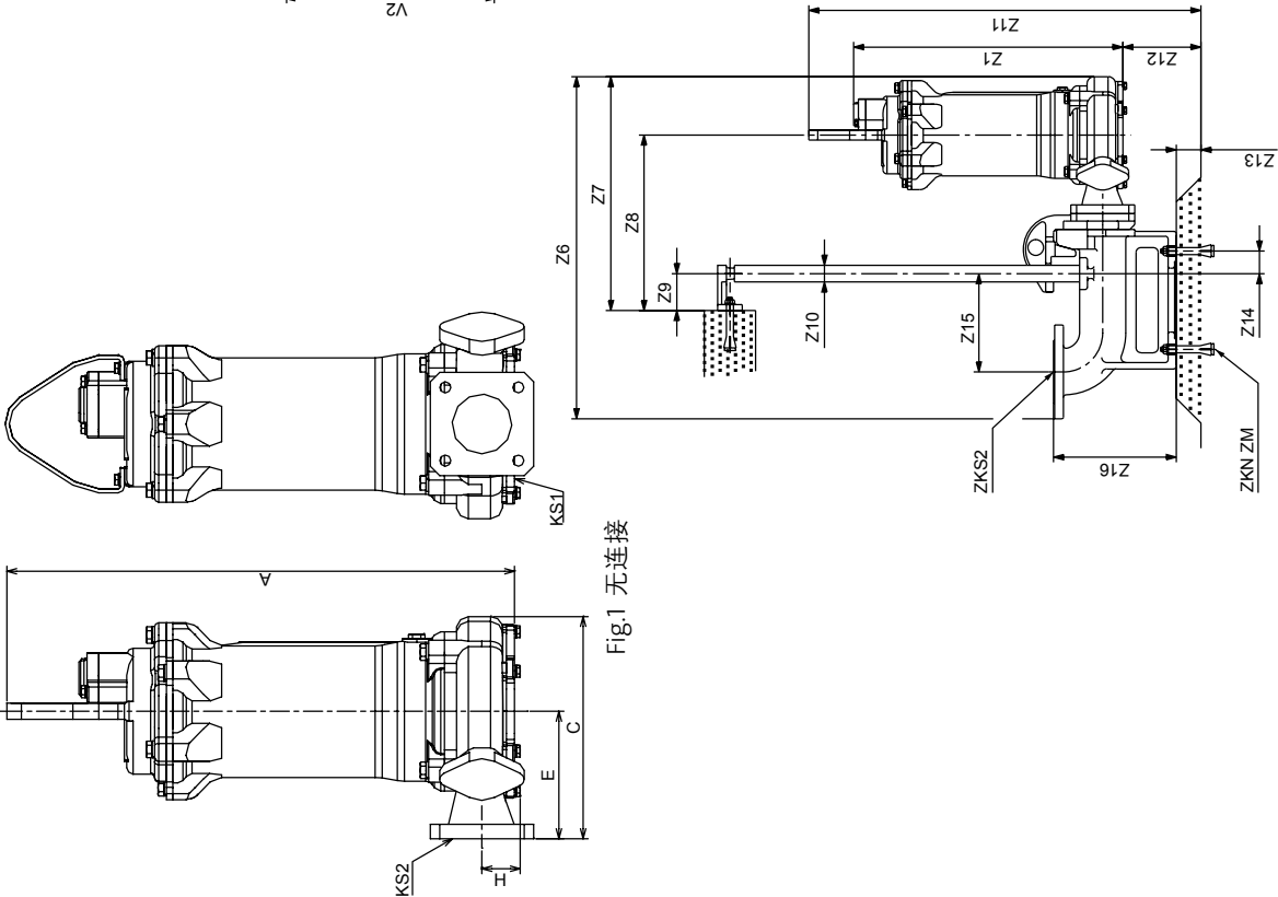
Fig.3 自耦连接
