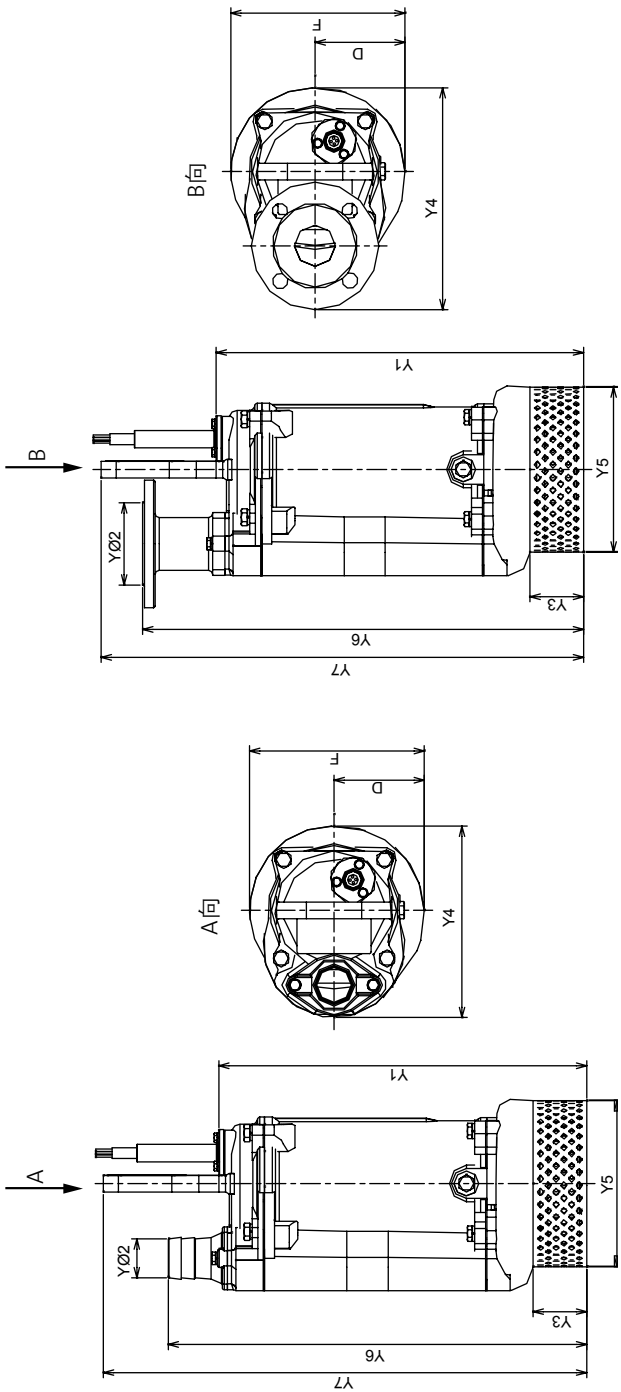
Fig.1 软管连接
